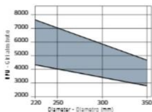
Minimum and maximum RPM based on the blade diameter. Fascia dei giri minimo e massimo consigliati in funzione del diametro della lama.
