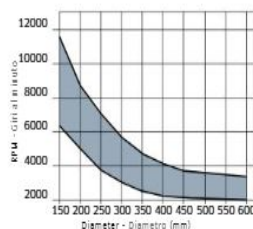
Minimum and maximum RPM based on the blade diameter. Pascio dei N. giri minimo e massimo consigliati in funzione del diametro della lama.
