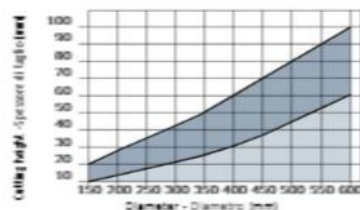
Maximum depth of rip and crosscut based on the blade diameter. Altezza di taglio lungo e traverso: valore massimo consentita in funzione del diametro della lama.
