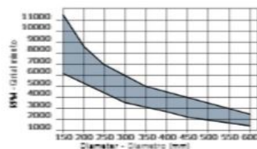
Minimum and maximum RPM based on the blade diameter. Scala dei R. giri minimo e massimo consigliati in funzione del diametro della lama.
