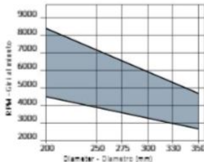
Minimum and maximum RPM based on the blade diameter. Fascia dei R. giri minimo e massimo consigliati in funzione del diametro della lama.
