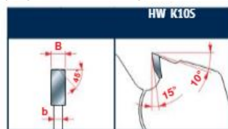
Tooth features - Caratteristiche del dente
