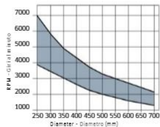
Minimum and maximum RPM based on the blade diameter. Fascie dei giri minimo e massimo consigliati in funzione del diametro della lama.
