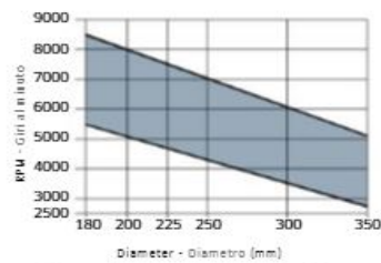
Minimum and maximum RPM based on the blade diameter. Pascia del N. giri minimo e massimo consigliati in funzione del diametro della lama.
