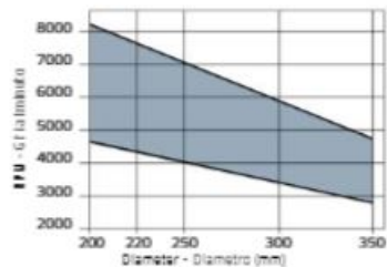
Minimum and maximum RPM based on the blade diameter. Fascia dei R. giri minimo e massimo consigliati in funzione del diametro della lama.
